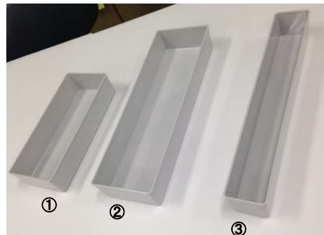
トレイインサート ①TI-211 ￥**** 外寸法/W242×D115×H51mm 内寸法/W220×D94×H49mm ②TI-311 ￥**** 外寸法/W345×D120×H51mm 内寸法/W322×D100×H49mm ③TI-35 ￥**** 外寸法/W342×D60×H51mm 内寸法/W322×D40×H49mm 材質/ABS(持続性帯電防止)
