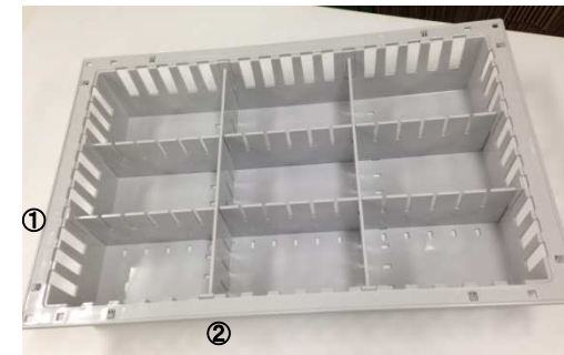
仕切板 ①PS-106 ￥**** 外寸法/W552×D17×H98mm ②PS-104 ￥*** 外寸法/W352×D17×H98mm ③PS-103 ￥*** 外寸法/W252×D17×H98mm ④PS-166 ￥**** 外寸法/W552×D17×H158mm ⑤PS-164 ￥**** 外寸法/W352×D17×H158mm
