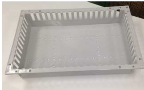
モジュラートレイ BAS-6410 ￥**** 外寸法/W600×D400×H108mm 内寸法/W535×D335×H102mm 材質/ABS(持続性帯電防止)
