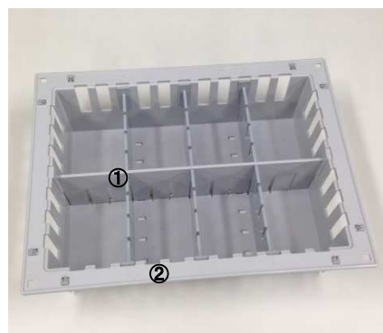
仕切板 ①PS-104 ¥*** 外寸法/W352×D17×H98mm ②PS-103 ¥*** 外寸法/W252×D17×H98mm 材質/ABS(持続性帯電防止)
